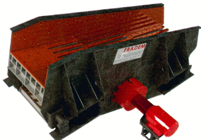
Crible Scalpeur FSI 52 Sovemat, Bourg d'Oisans (Isère)
